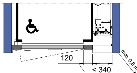
PIANTA PIANO GRUPPO DI MANOVRA TELAIO PORTE MRF 120 (STANDARD ED EI120)
