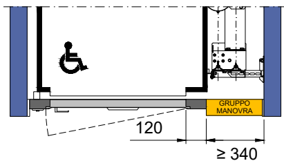
PIANTA PIANO GRUPPO DI MANOVRA TELAIO PORTE MRF 120 (STANDARD ED EI120)
