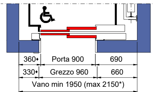
PIANTA VANO CORSA TELAIO PORTE NF (EI120)
