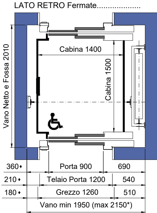
PIANTA VANO CORSA TELAIO PORTE MRF 150
