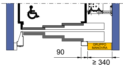
PIANTA PIANO GRUPPO DI MANOVRA TELAIO PORTE MRF 90 (STANDARD ED EI120)
