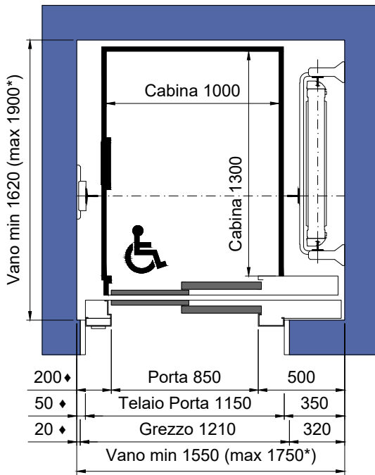
PIANTA VANO CORSA TELAIO PORTE MRF 150
