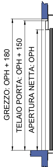
SEZIONE TELAIIO PORTE MRF 150
