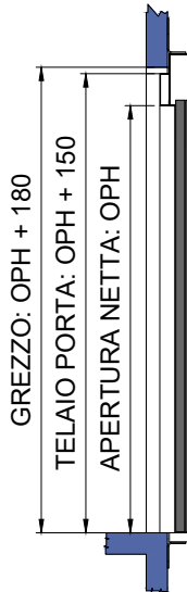
SEZIONE TELAIO PORTE MRF 150
