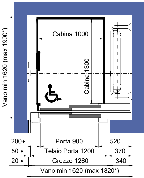
PIANTA VANO CORSA TELAIO PORTE MRF 150
